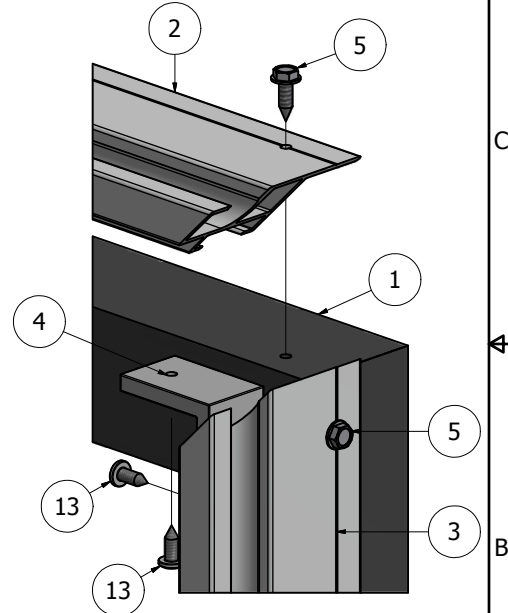
DETAIL A-2
